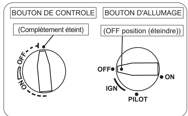
Fig. 51-2 Arrêt manuel
