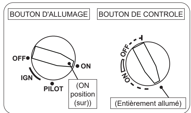
Fig. 51-1 Éclairage manuel
